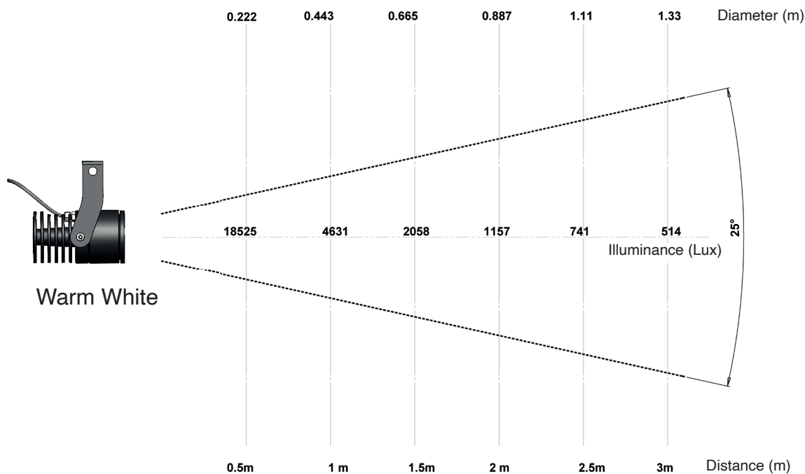
Lexys U-BRACKET 3000K 25°
