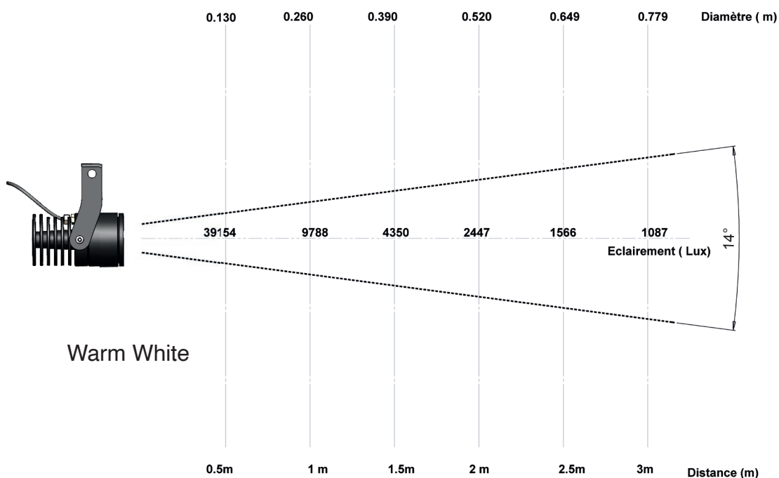
Lexys U-BRACKET 3000K 14°
