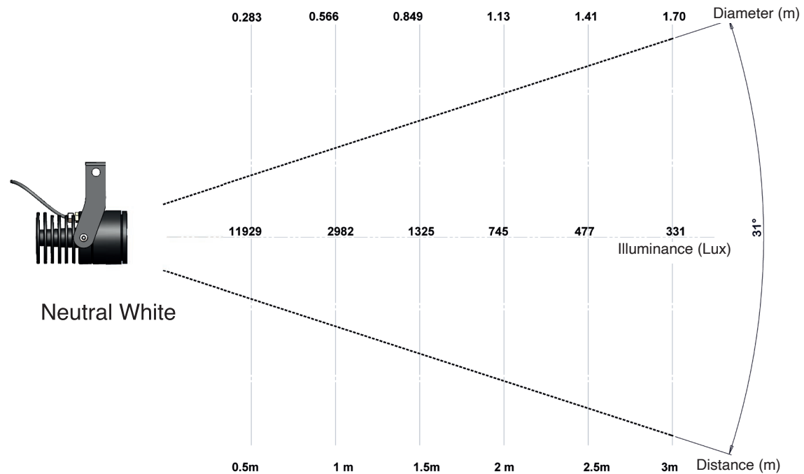
Lexys U-BRACKET 4000K 31°
