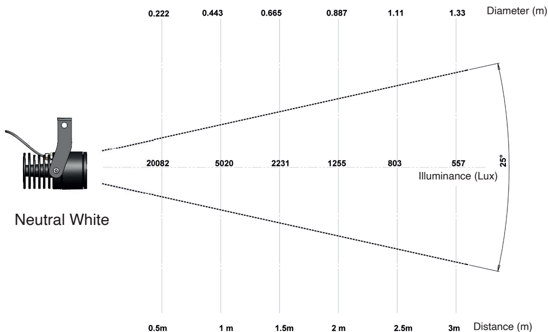
Lexys U-BRACKET 4000K 25°
