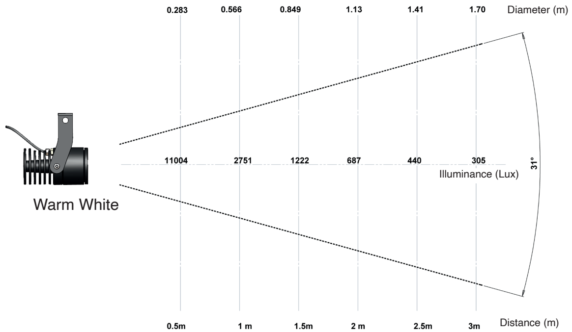
Lexys U-BRACKET 3000K 31°
