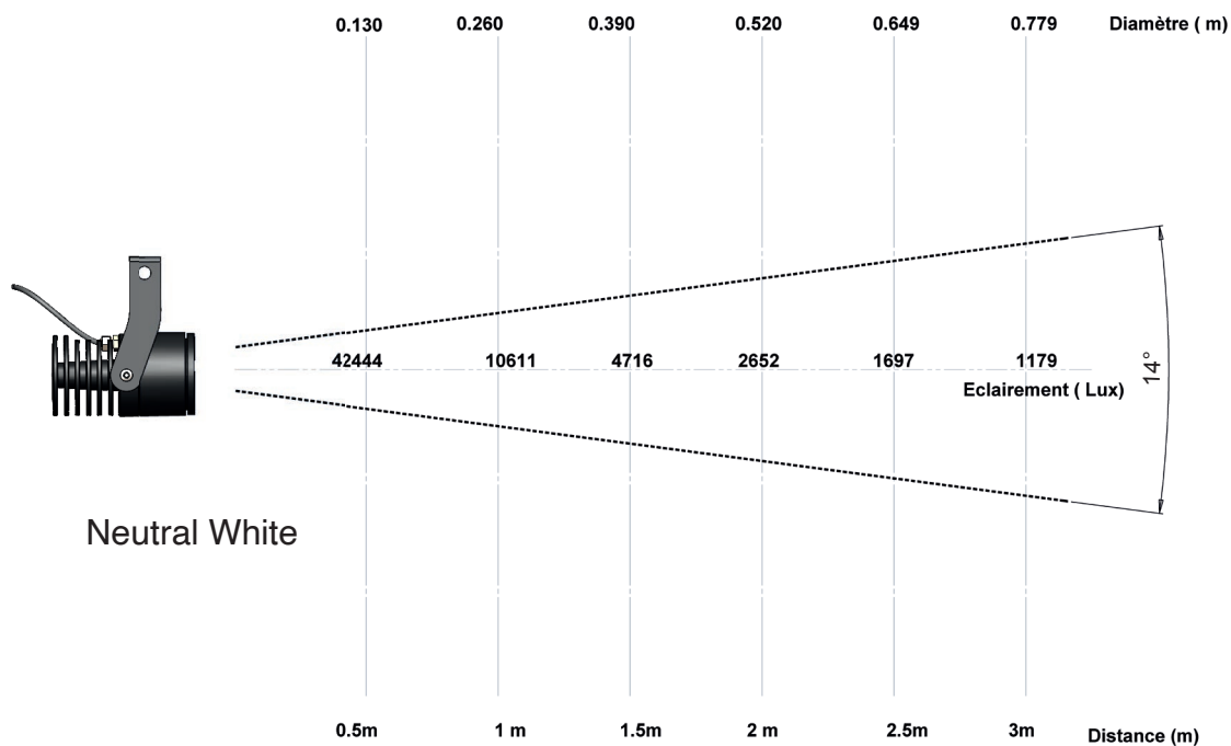
Lexys U-BRACKET 4000K 14°
